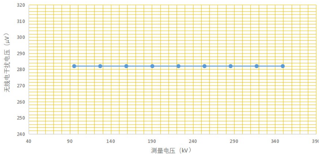
无线电干扰测量曲线
