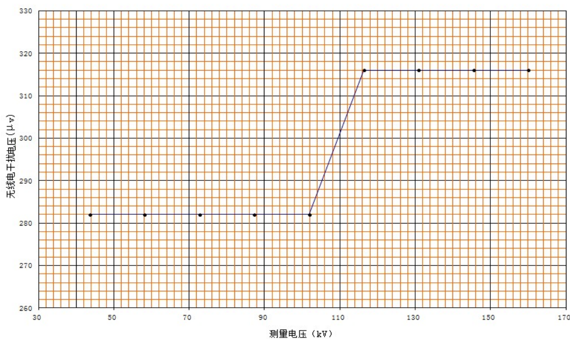
无线电干扰测量曲线
