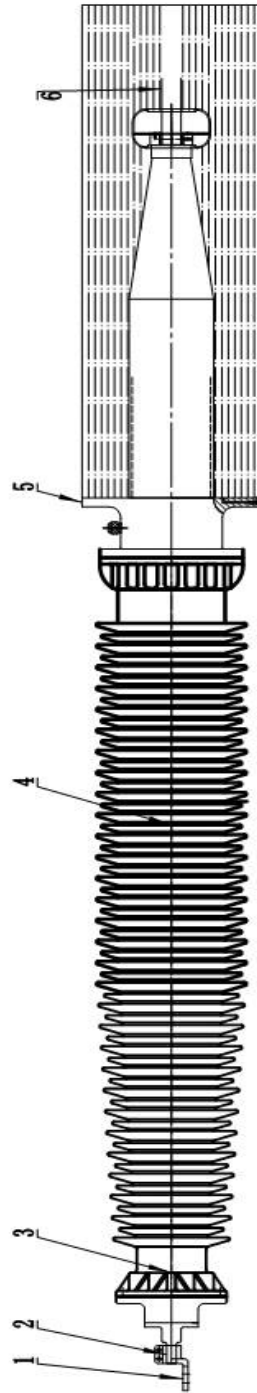
套管升温测量点位置示意图
