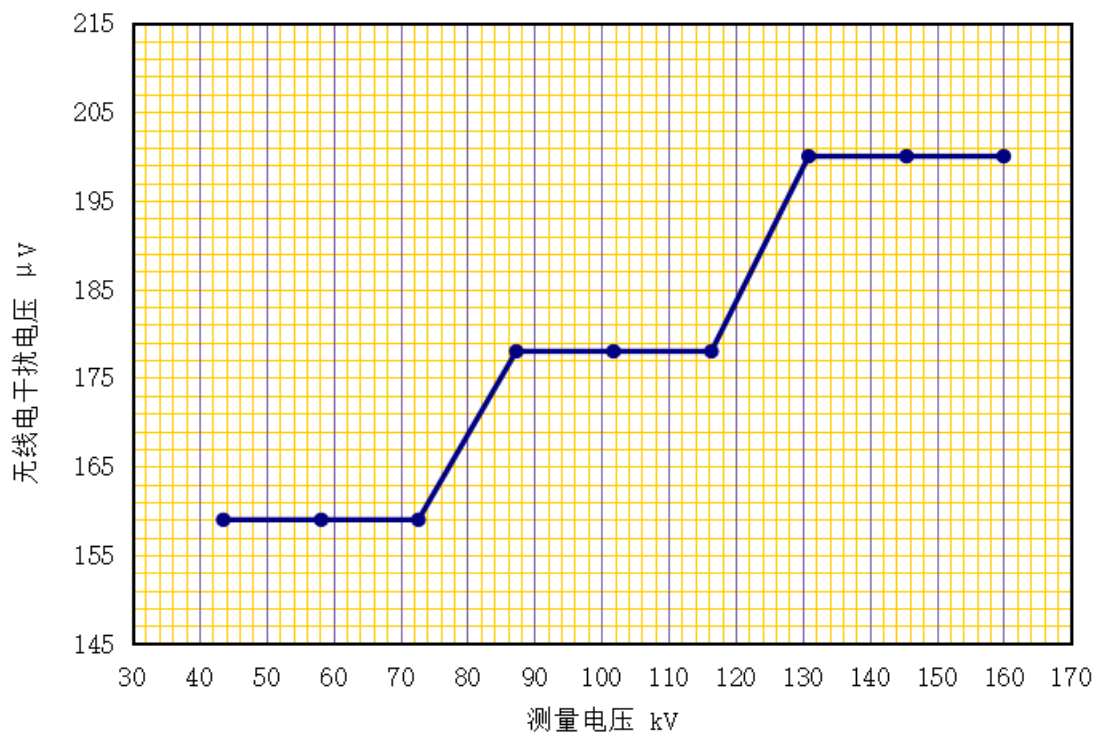
无线电干扰测量曲线
