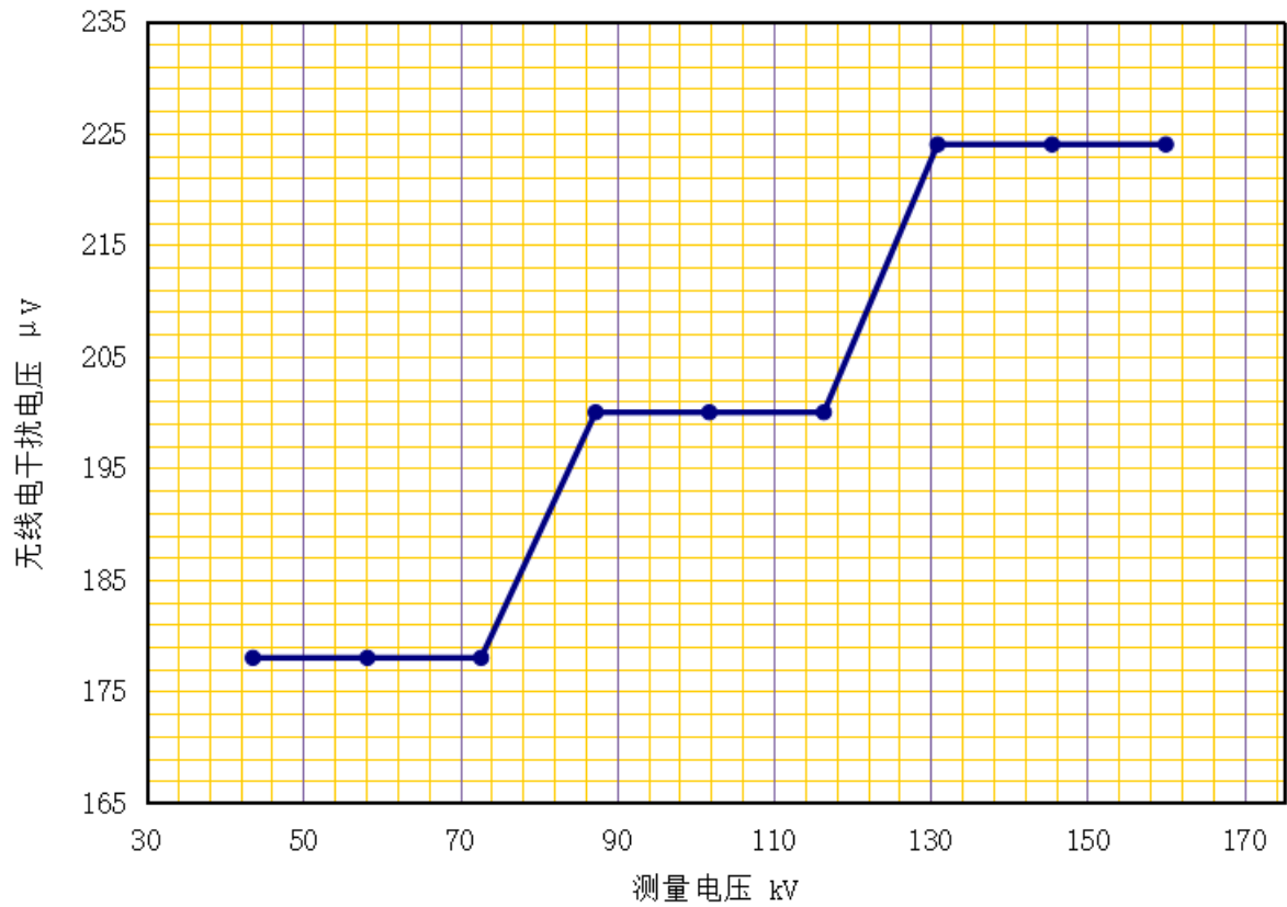
无线电干扰测量曲线
